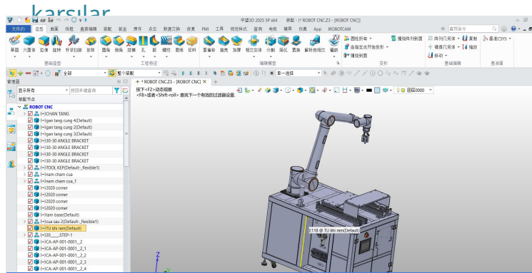
Bileşik Robot Tasarımı
